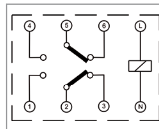
ANSCHLUSS Anschlussschema
